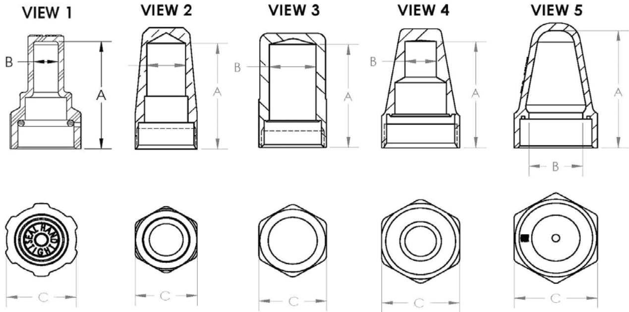
Dimensions
